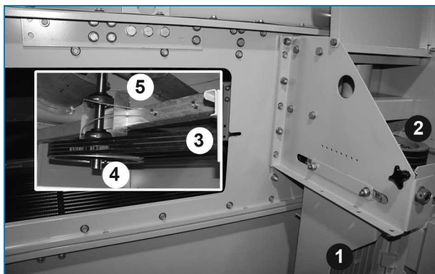
Drivsystem med yttre motor
