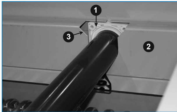
BranchLok™ demonterbart spraystem
