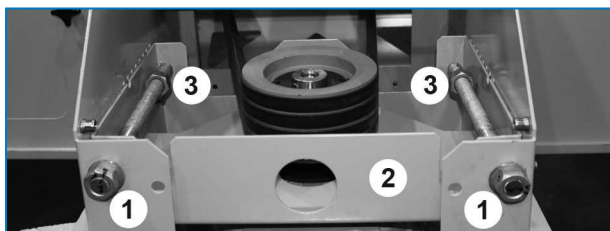
Justerbar motorbas
