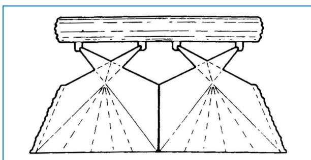
Vattenfördelningsbild från dysorna på kyltorn
