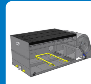
Патрубки очистки поддона
