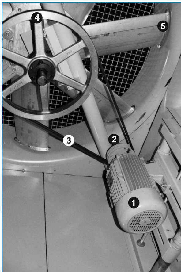
Hajtóműrendszer
