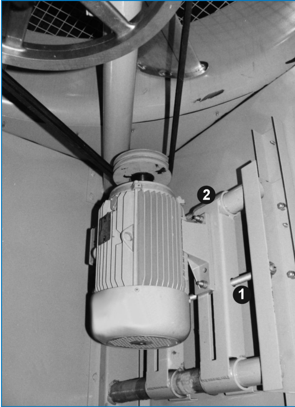
Igazítható motoralap
